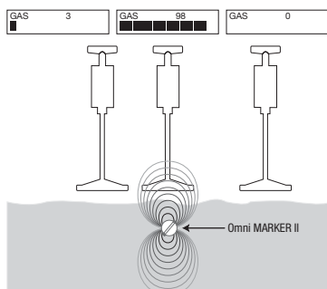
Abbildung 22. Omni Marker II Signal
