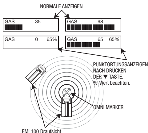
Abbildung 14. Punktortungsfunktion
