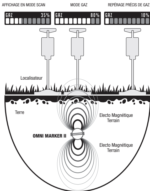
Figure 15. Exemples de modes d'affichage
