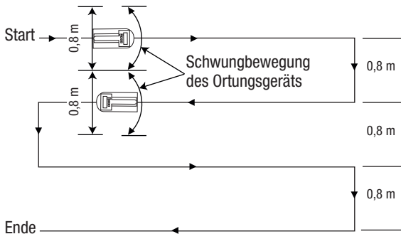
Abbildung 16. Suchmuster
