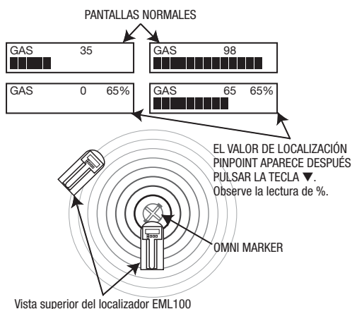
Figura 14. Característica Pinpoint
