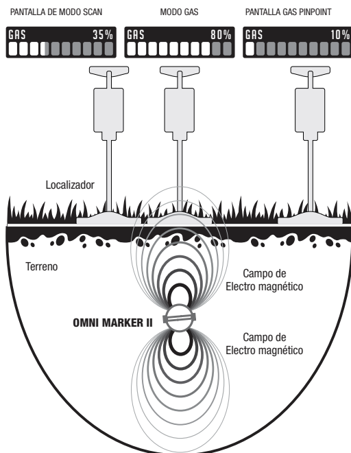
Figura 15. Ejemplos de pantallas de modo
